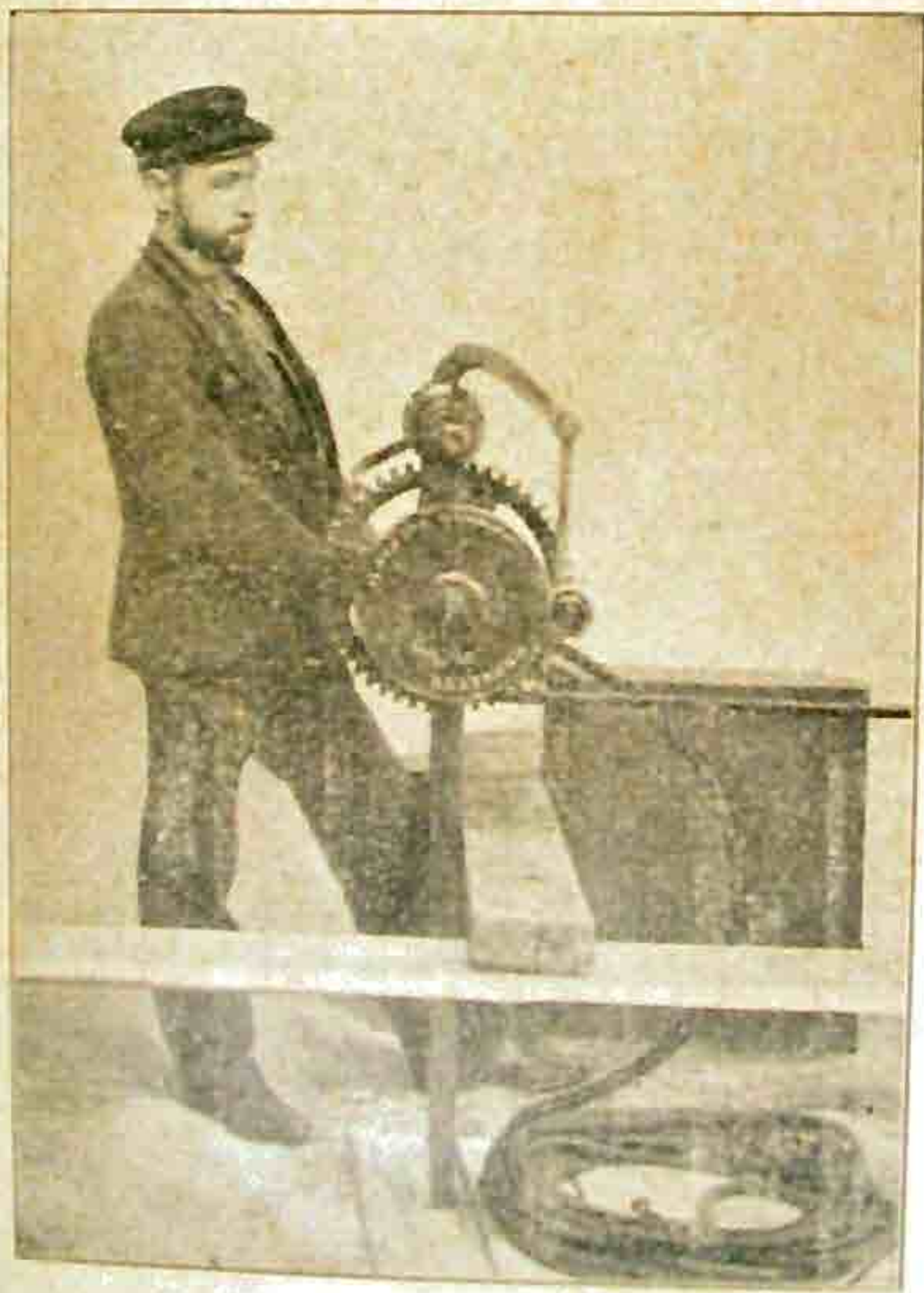
Patenteret Not- og Kabelspil.
