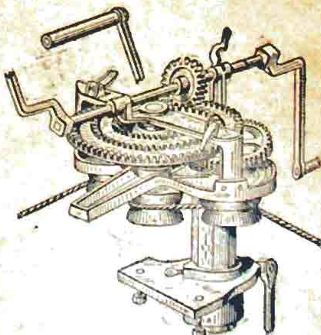
Patenteret Garnspil
