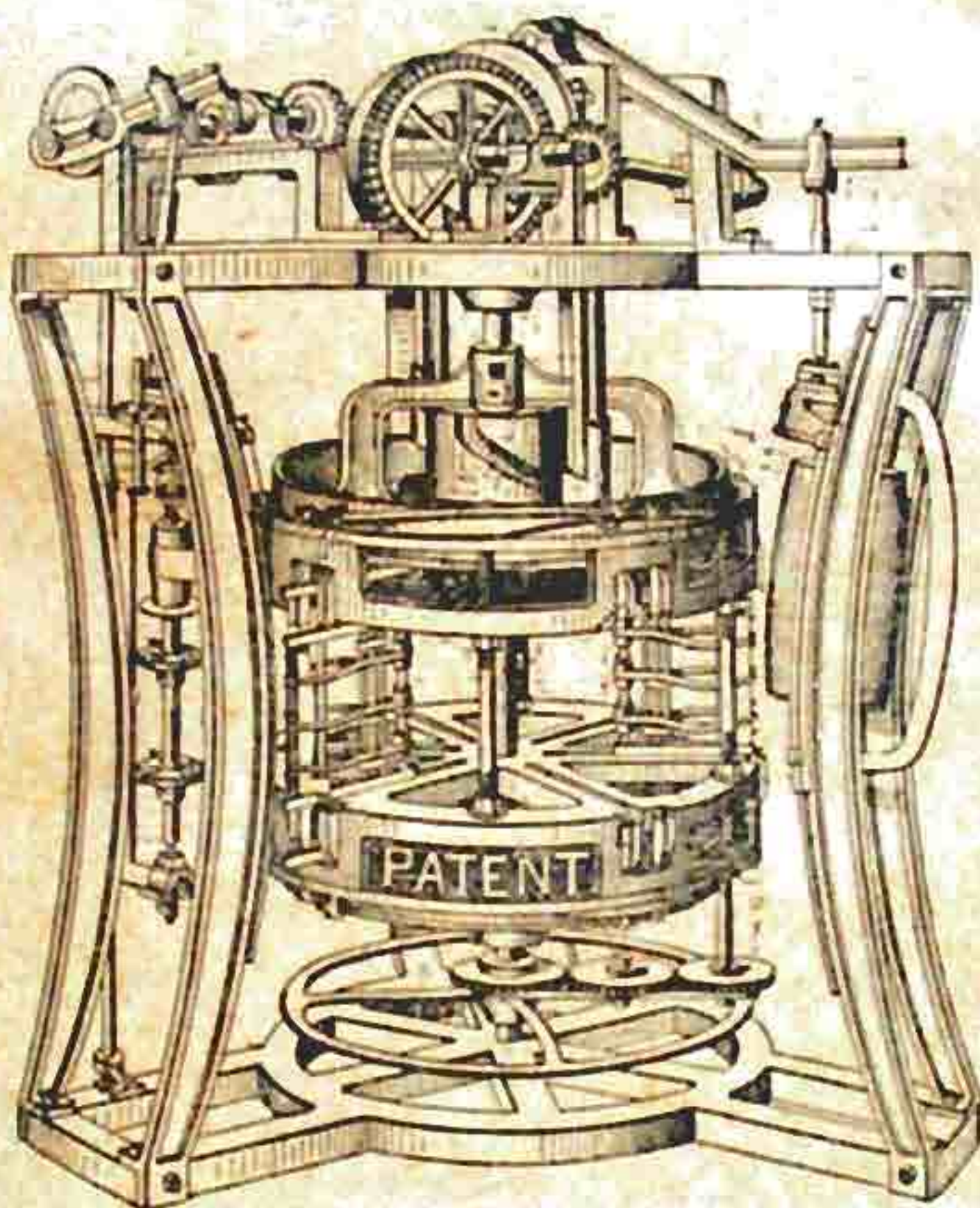
Patenteret Tøndestavmaskine
